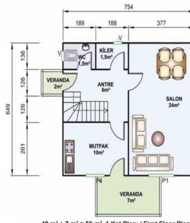
49 m 2 + 7 m 2 = 56 m 2 1.Kat Planı / First Floor Plan
