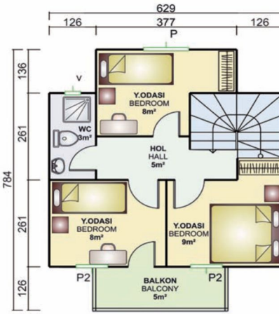
38 m 2 + 5 m 2 = 43 m 2 1.Kat Planı / First Floor Plan
