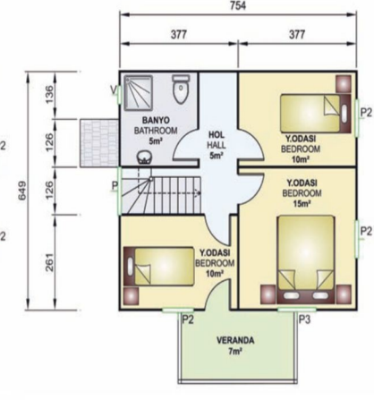
49 m 2 + 7 m 2 = 56 m 2 1.Kat Planı / First Floor Plan
