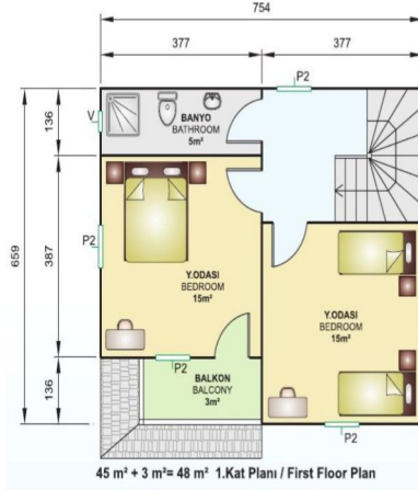
45 m 2 + 3 m 2 = 48 m 2 1.Kat Planı / First Floor Plan
