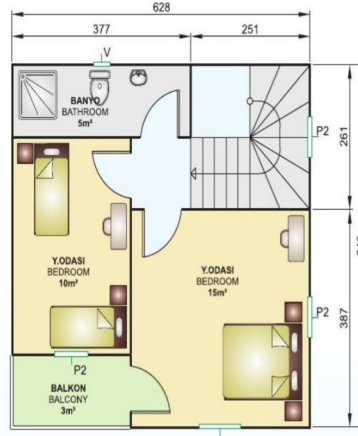
37 m 2 + 3 m 2 = 40 m 2 1.Kat Planı / First Floor Plan
